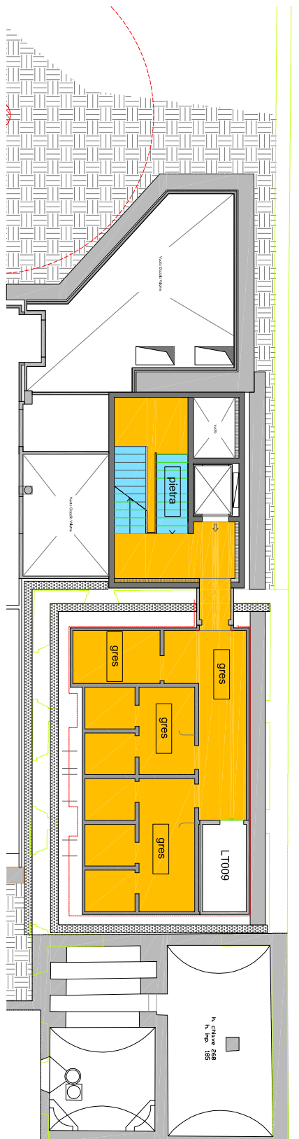
PIANO TERRA Quota -3,58 scala 1:200
