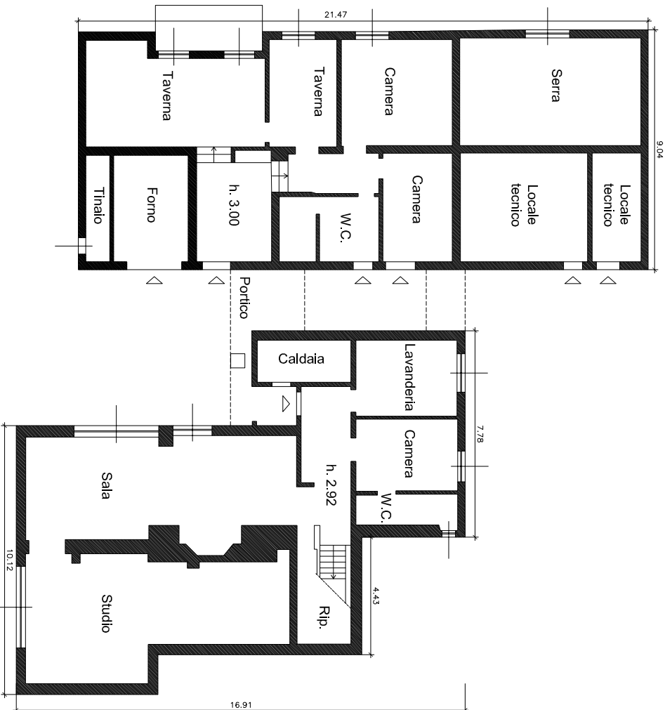
PIANO TERRA scala 1:200
