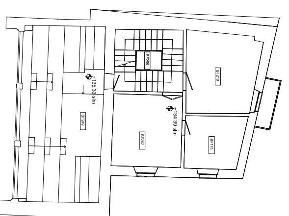
PIANO QUARTO INFERIORE Quota 135.33 slm scala 1:200
